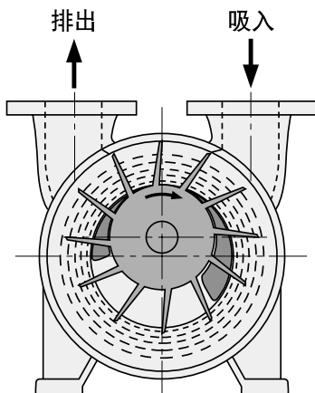
水封真空泵
